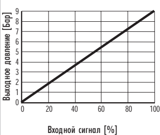
РЕГУЛИРОВОЧНАЯ ХАРАКТЕРИСТИКА ER-2XX-9XXX
